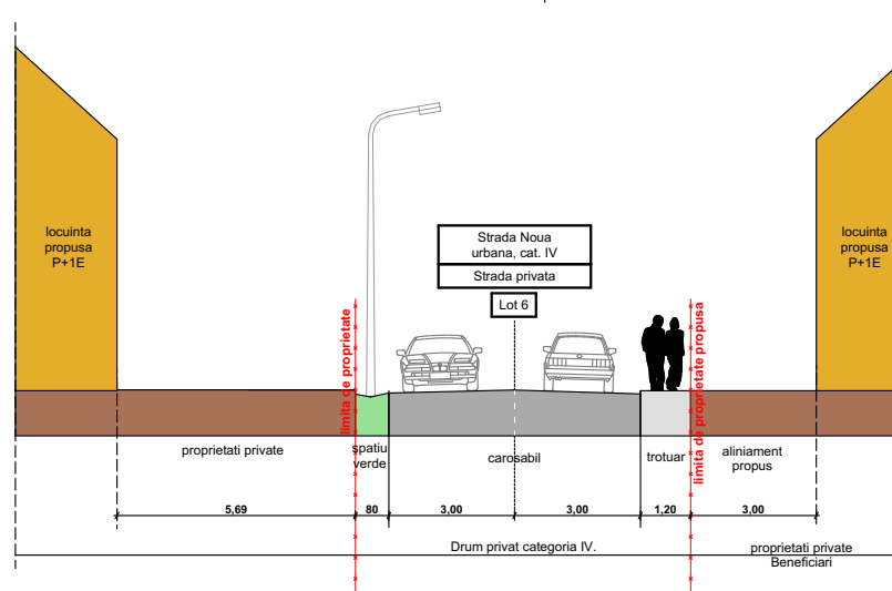
PROFIL STRADAL B-B - strada noua propusa
