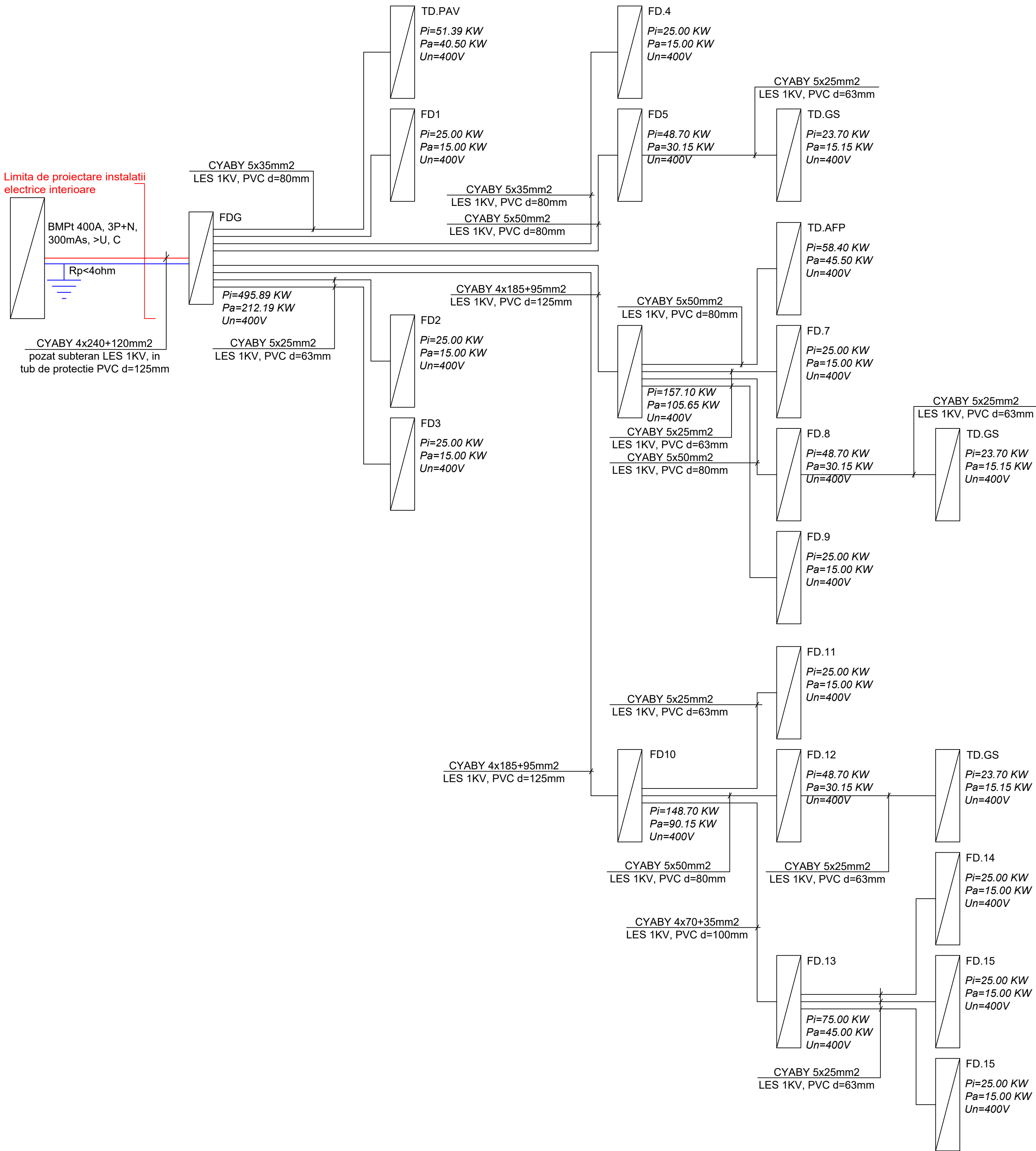
Schema monofilara de distributie generala
