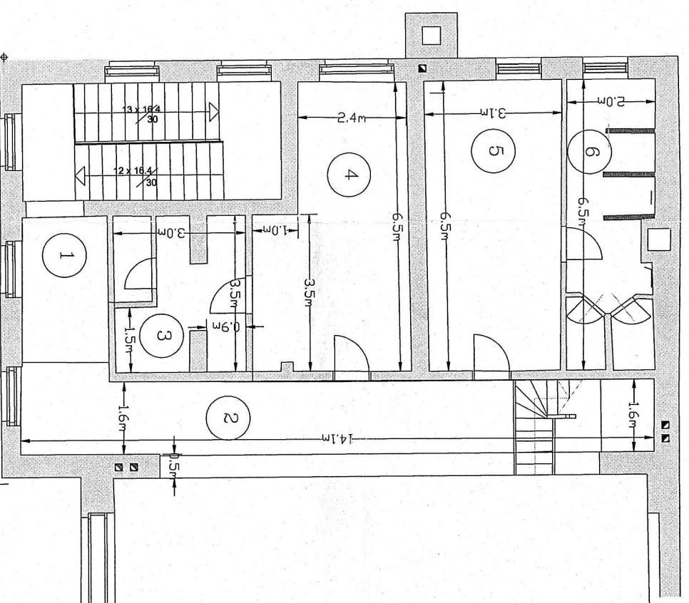
C8 - Plan etaj
